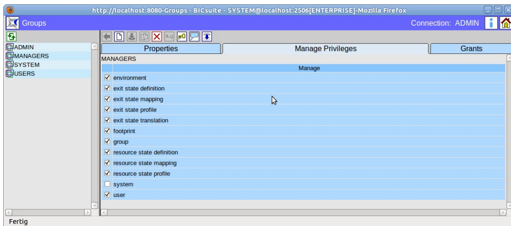
Abbildung 17.3: Manage Privilegien einer Gruppe
