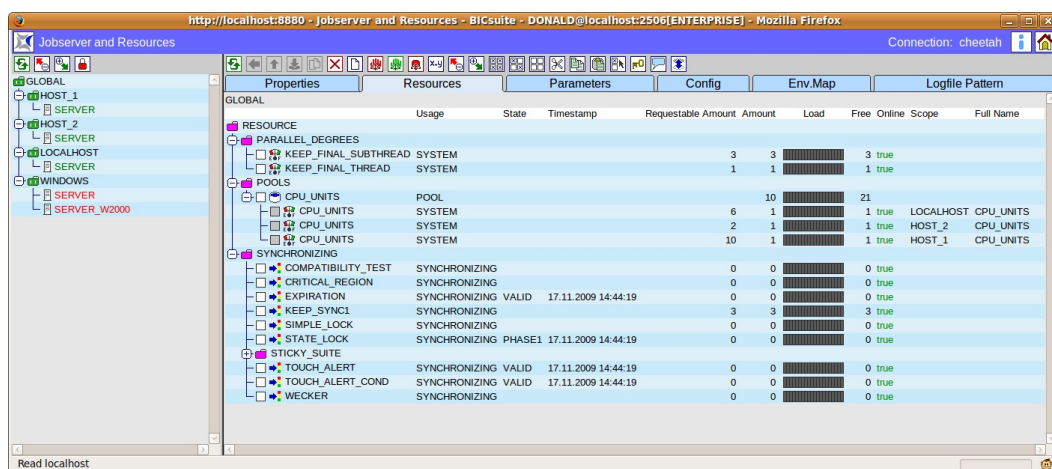
Abbildung 13.5: Jobserver und Scope Ressourcen
