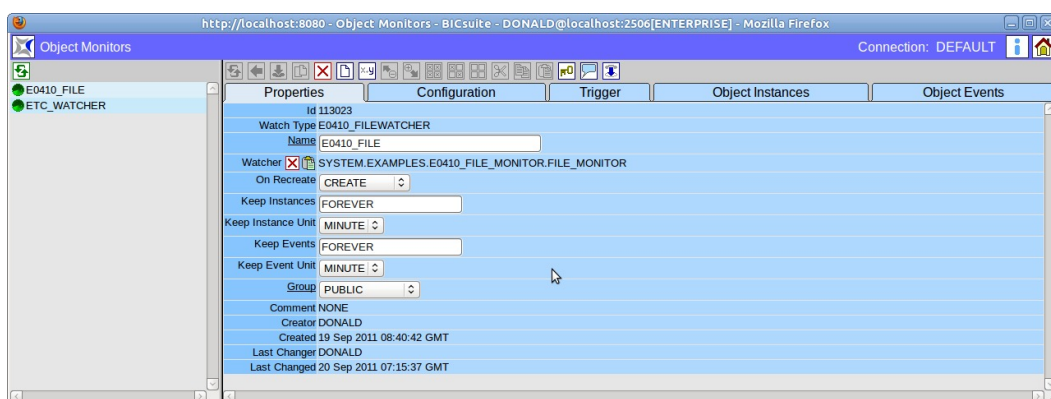
Abbildung 25.4: Object Monitoring Eigenschaften
