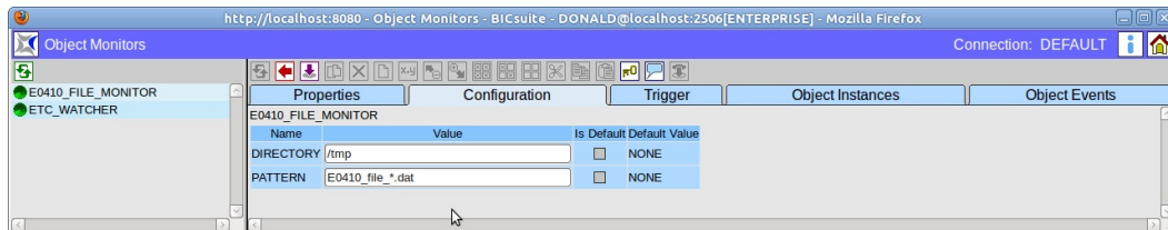
Abbildung 25.5: Object Monitoring Konfiguration
