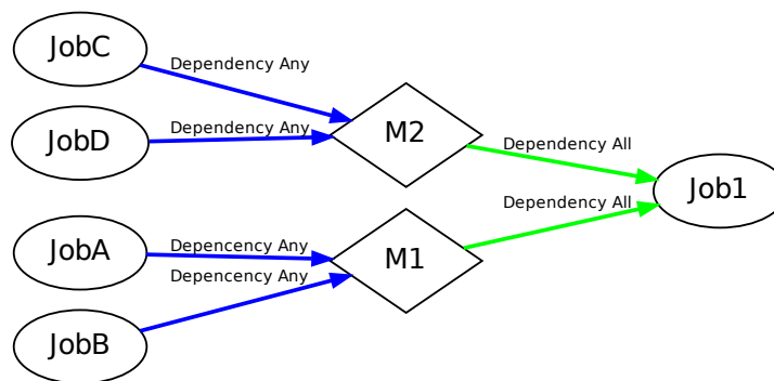
Abbildung 14.22: Beispiel für Dependency Modes
