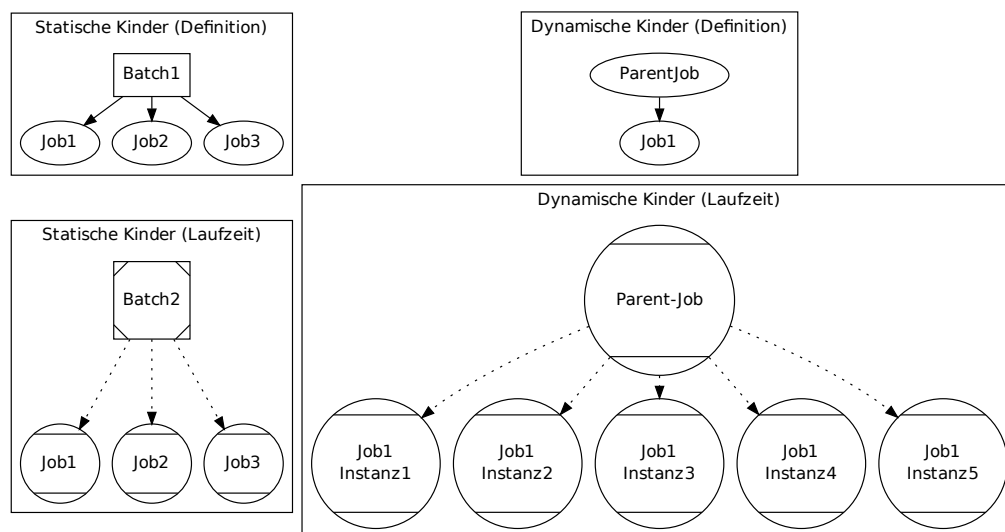
Abbildung 14.17: Statische und dynamische Children
