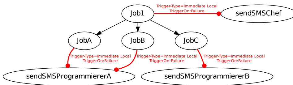
Abbildung 14.38: Beispiel für Immediate Local Trigger
