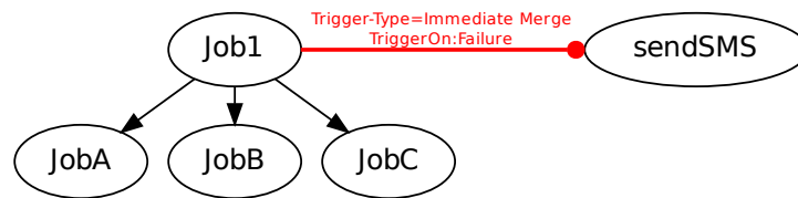
Abbildung 14.37: Beispiel für Immediate Merge Trigger
