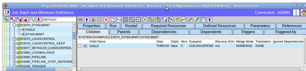
Abbildung 14.15: Batches und Jobs; Children Tab
