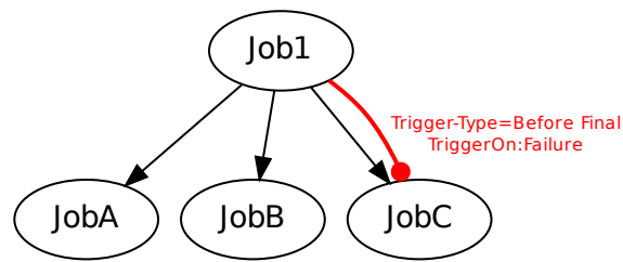
Abbildung 14.39: Beispiel für Before Final Trigger
