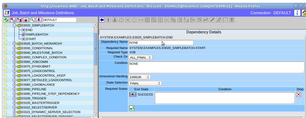
Abbildung 14.23: Batches und Jobs; Dependency Details
