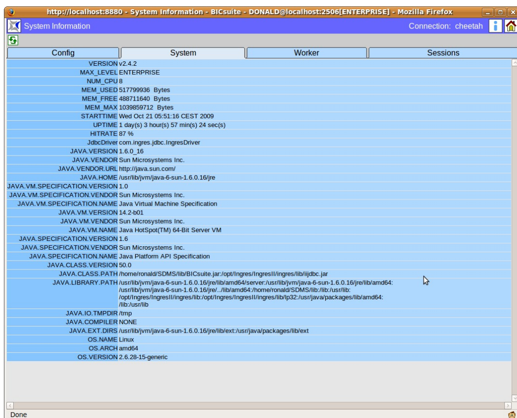
Abbildung 24.3: System Runtime Umgebung
