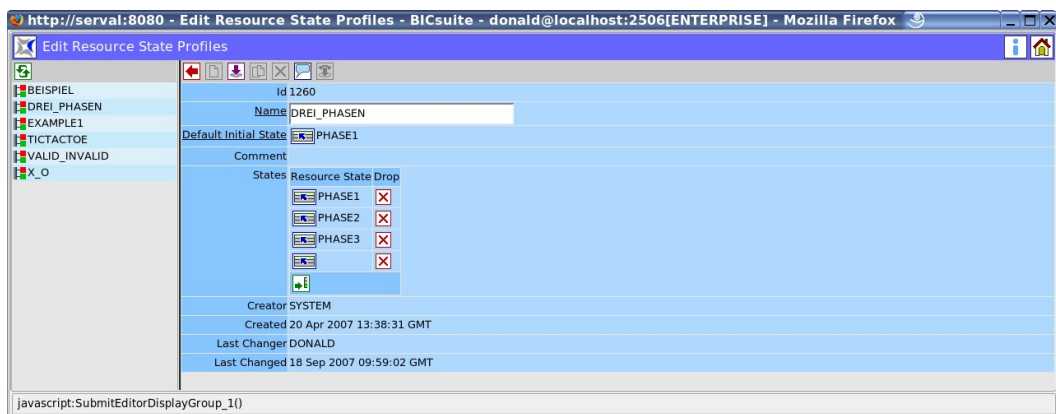
Abbildung 1.22: Listen Handling; Zufügen einer Zeile
