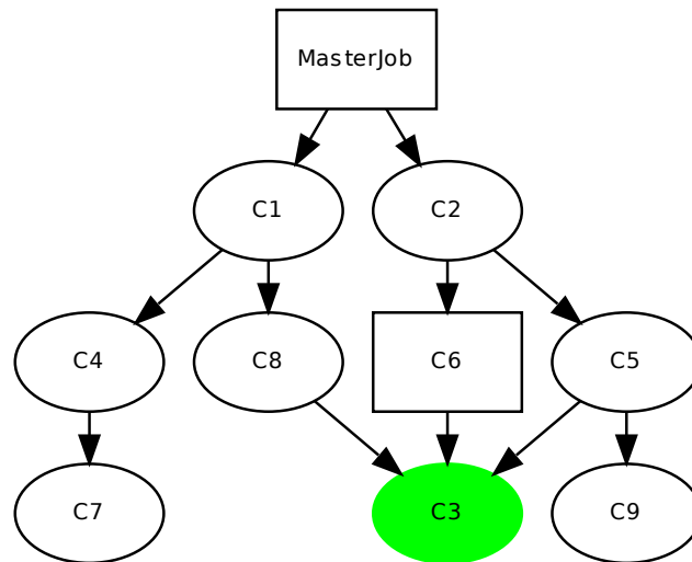
Abbildung 14.18: Beispiel für Merge Mode
