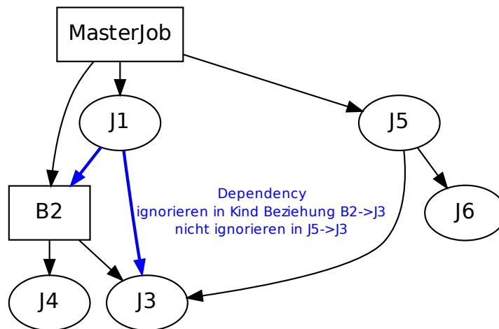
Abbildung 14.19: Beispiel Ignored Dependencies
