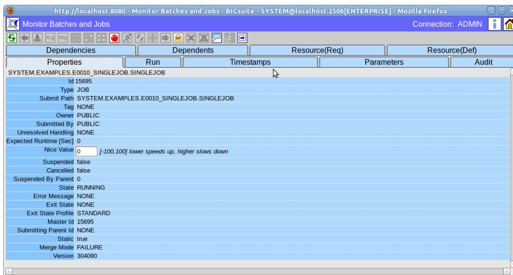
Abbildung 21.9: Job und Batch Properties
