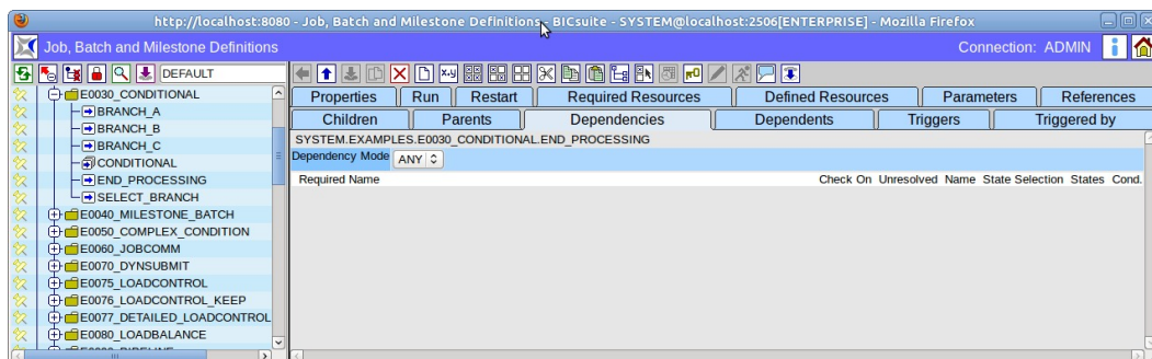
Abbildung 1.34: Verknüpfen von Objekten; Anfangssituation
