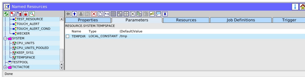
Abbildung 10.5: Named Resources; Parameter Tab
