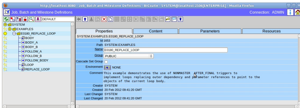
Abbildung 14.4: Batches und Jobs; Ansicht mit Pin
