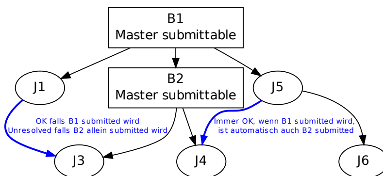
Abbildung 14.24: Beispiel für Unresolved Handling
