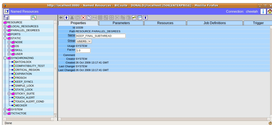
Abbildung 1.9: Suchen im Navigator
