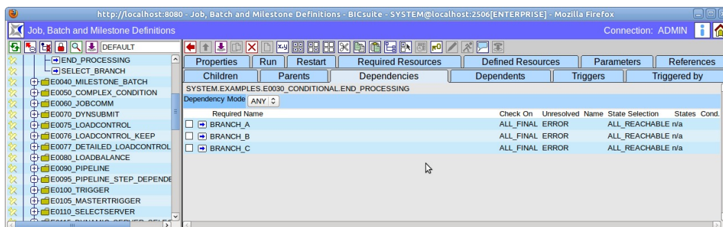
Abbildung 1.36: Verknüpfen von Objekten; Einfügen
