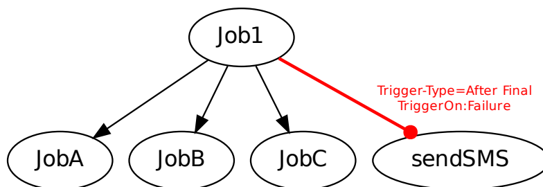
Abbildung 14.40: Beispiel für After Final Trigger
