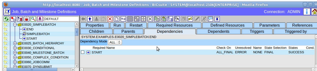
Abbildung 14.21: Batches und Jobs; Dependencies Tab
