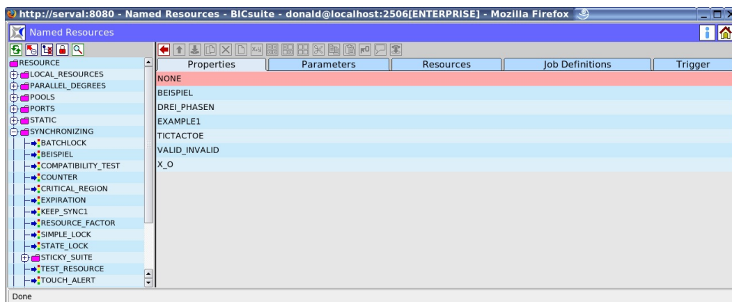
Abbildung 1.19: Auswahl eines Resource State Profiles; Auswahlliste
