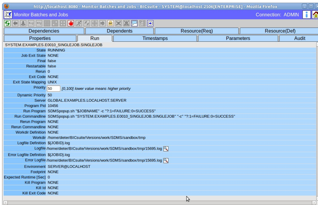
Abbildung 21.10: Batch und Job Run Information
