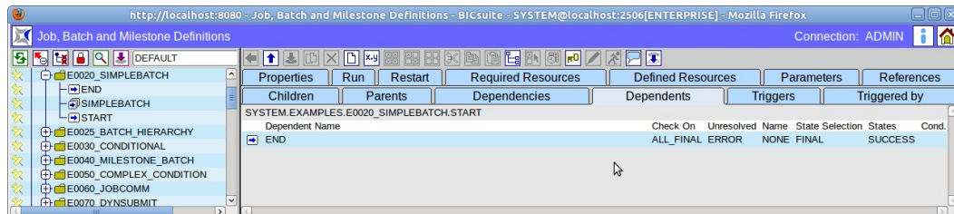
Abbildung 14.25: Batches und Jobs; Dependents Tab
