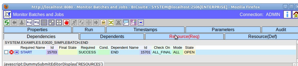
Abbildung 21.12: Batch und Job Abhängigkeiten
