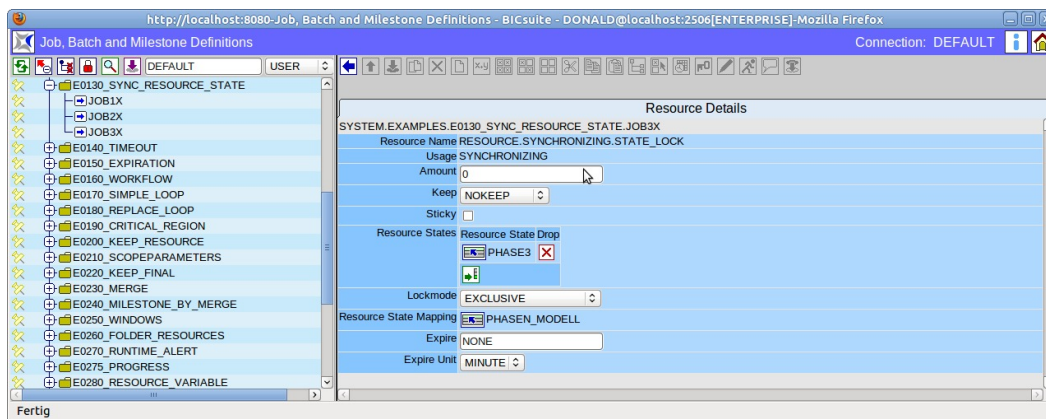
Abbildung 14.27: Batches und Jobs; Resource Requirement Details
