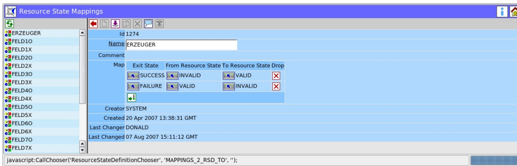
Abbildung 8.2: Resource State Mapping Beispiel
