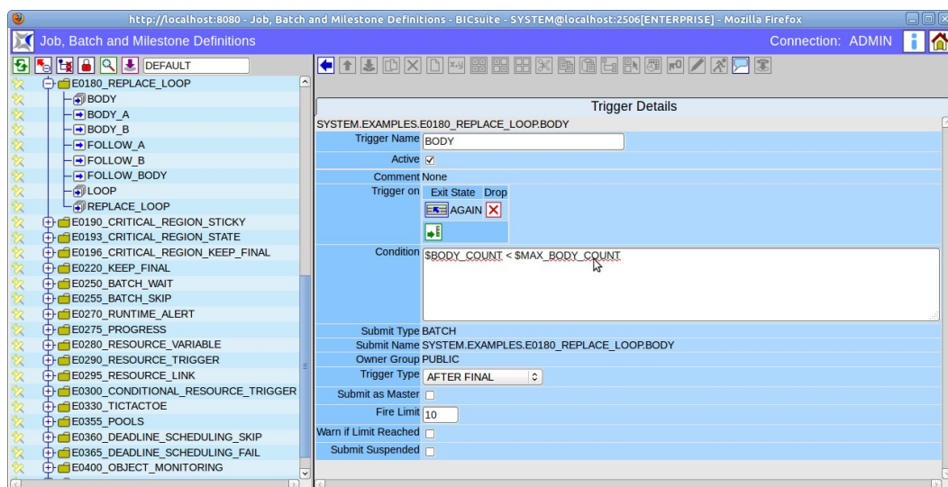
Abbildung 14.36: Batches und Jobs; Trigger Details
